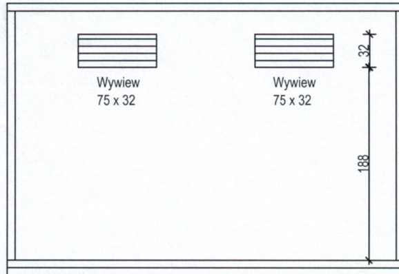
Elewacja południowa
